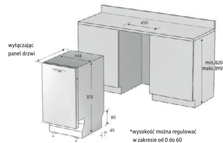
Rysunek techniczny dotyczy modeli: DW50K4050BB, DW50K4030BB
