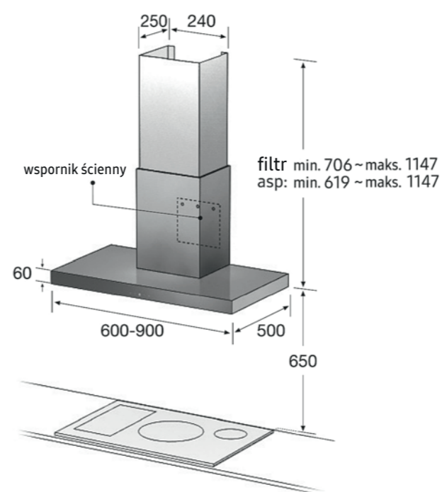
Rysunek techniczny dotyczy modeli: NK36M5070BG, NK24M5070BG
