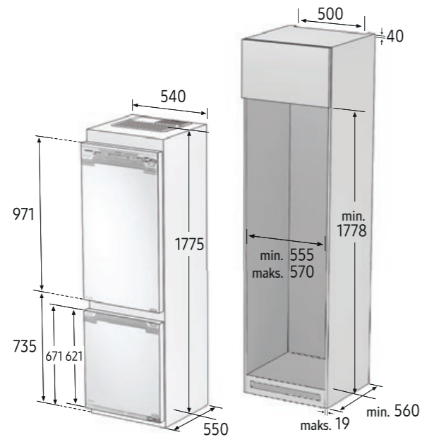
Rysunek techniczny dotyczy modelu: BRB260187WW
