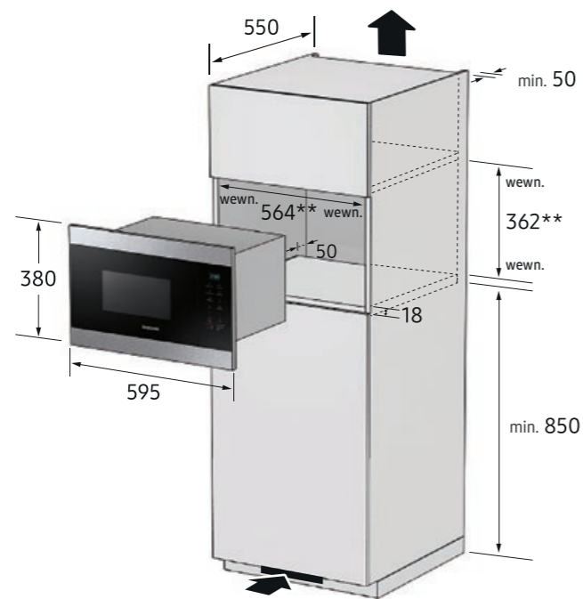
Rysunek techniczny dotyczy modeli: MG22M8074AT, MG22M8054AK, MS22M8054AK
