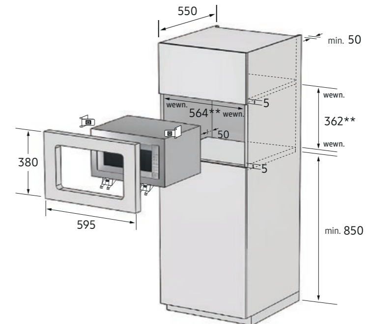
Rysunek techniczny dotyczy modeli: FG87SUST, FG87SUB, FW87SUST, FW87SUB
