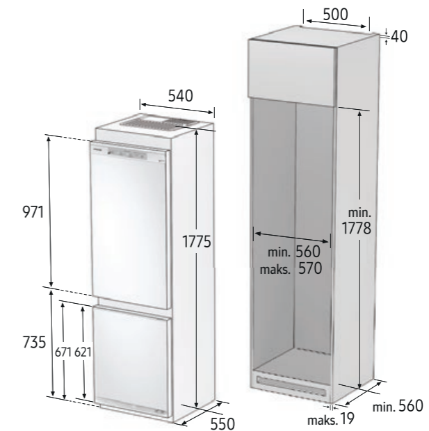
Rysunek techniczny dotyczy modeli: BRB260087WW, BRB260076WW, BRB260034WW, BRB260030WW, BRB260010WW
