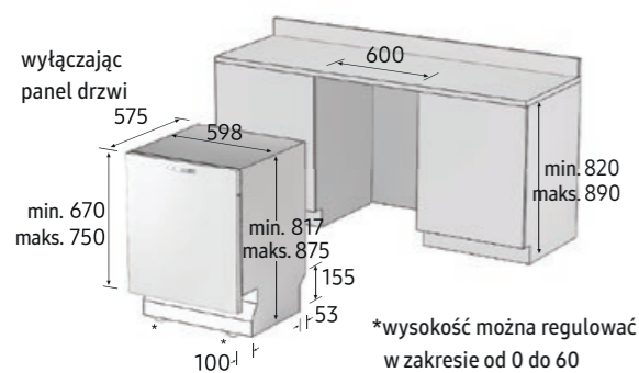
Rysunek techniczny dotyczy modelu: DW60K8550BB
