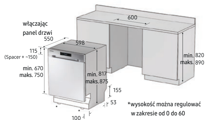
Rysunek techniczny dotyczy modelu: DW60M6040SS
