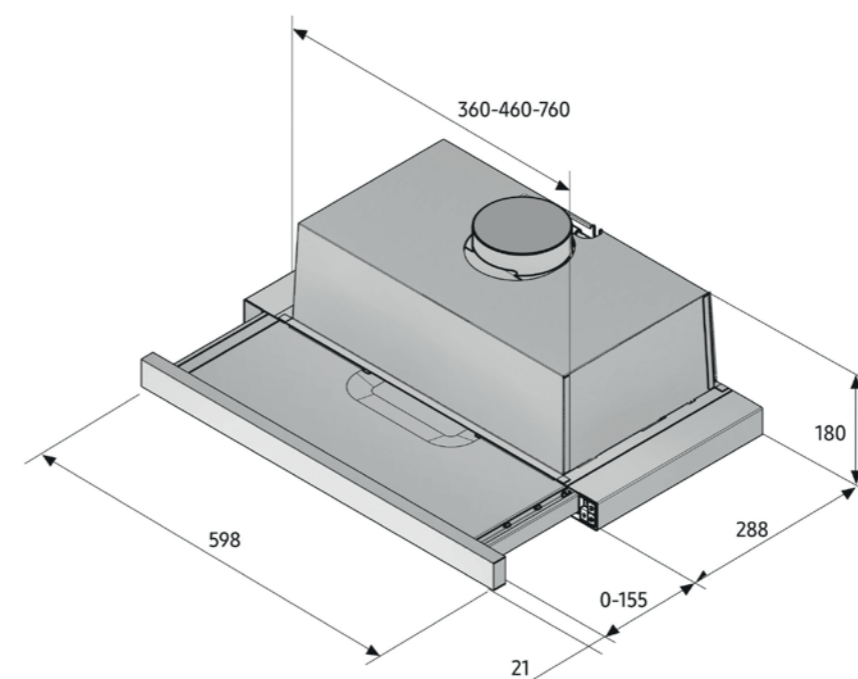
Rysunek techniczny dotyczy modelu: DW02034
