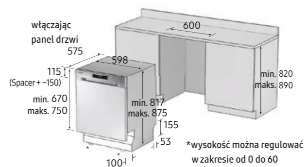
Rysunek techniczny dotyczy modelu: DW60M6050SS
