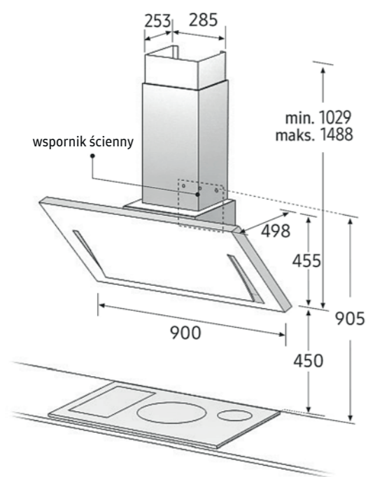
Rysunek techniczny dotyczy modelu: NK86NOV9MSR
