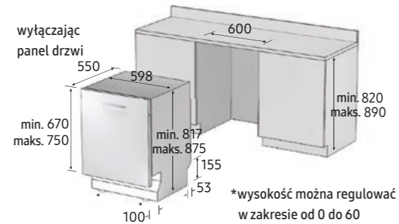
Rysunek techniczny dotyczy modeli: DW60M6050BB, DW60M6040BB, DW60M5060BB, DW60M5040BB
