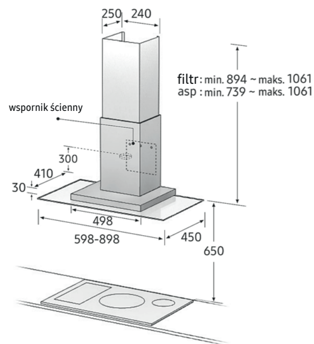
Rysunek techniczny dotyczy modeli: NK36M5070FS, NK24M5070FS
